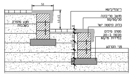
טריבונה על גבי טרסות מבלוקי קיסטון
