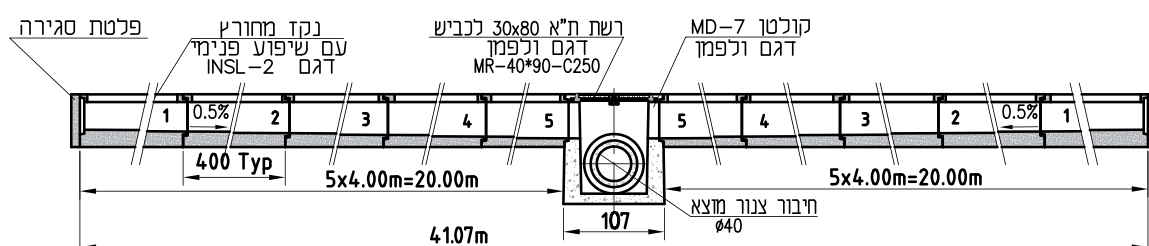
קטע נקזים מחורצים עם שיפוע פנימי (INSL) מתחבר אל קולטן MD-7, חתך אורכי. ק"מ - 1:75.
