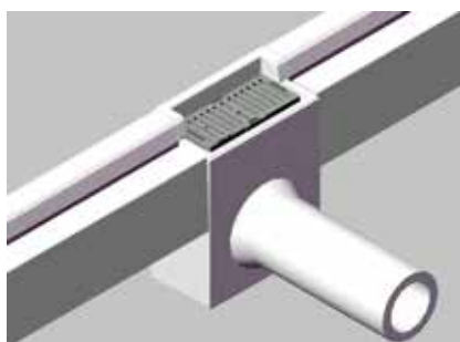
ועם אבן אי (פרופיל 2I) למערכת ניקוז ראשית באמצעות קולטן MD-7 וצינור בטון Ø 40
