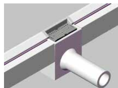
חיבור נקזים מחורצים עם אבן שפה (פרופיל 2K)
