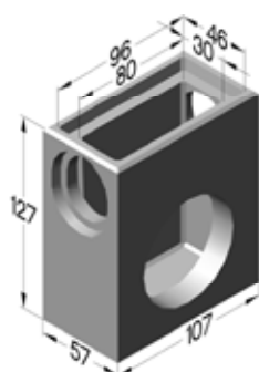
קולטן דגם MD-7 עם פתחי כניסה אובליים מתאימים לחיבור קטעי נקזים מחורצים בשני צדדי הקולטן
