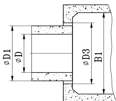
חיבור צינור ללא פעמון (צינור מנוסר) חיבור ע"י אטם קונטור סיל או חיבור ע"י טיט בטון + עוצר מים או חיבור ע"י טיט בטון בלבד
