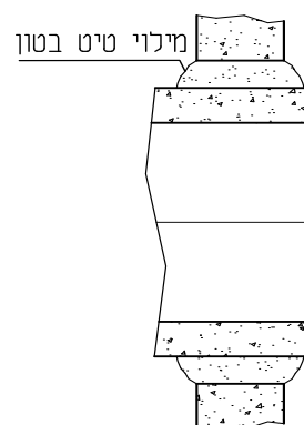
חיבור ע"י טיט בטון בלבד
