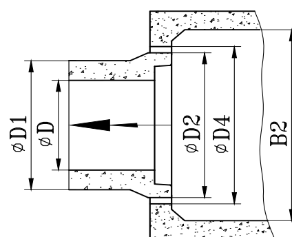
חיבור צינור עם פעמון
