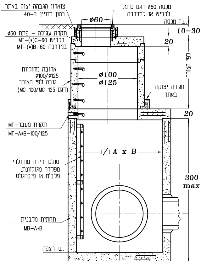
תא בקרה מלבני גדול עם ארובה
