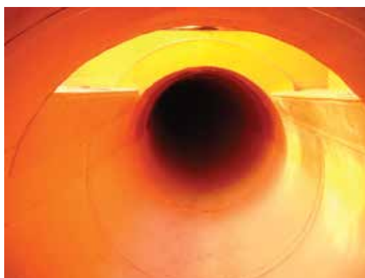
תא בקרה מלבני עם ציפוי ליינר HDPE בתשתית המטרופוליטית - גשר פז, חיפה
