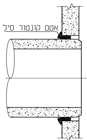
חיבור ע"י אטם קונטור סיל
