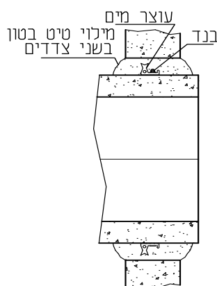
חיבור ע"י טיט בטון + עוצר מים
