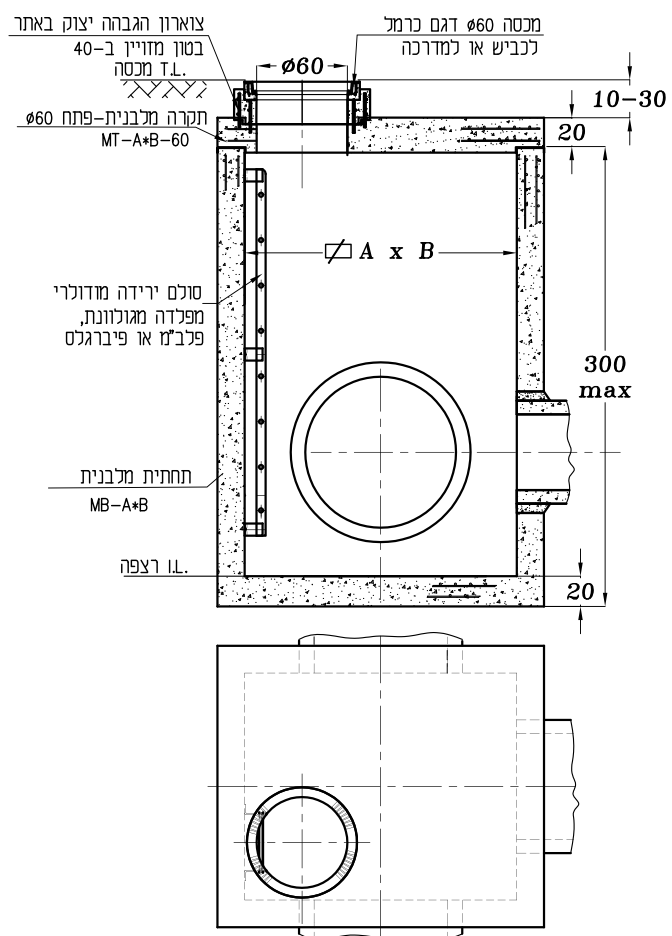
תא בקרה מלבני גדול עם תקרה
