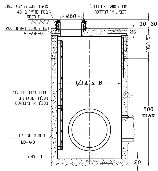
תא בקרה מלבני גדול עם תקרה
