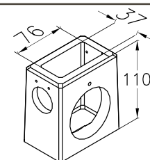
קולטן ראשי לרשת ללא אבן שפה
