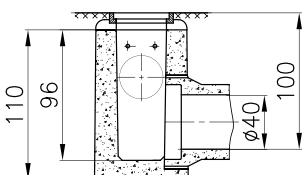
קולטן ראשי לרשת ללא אבן שפה
